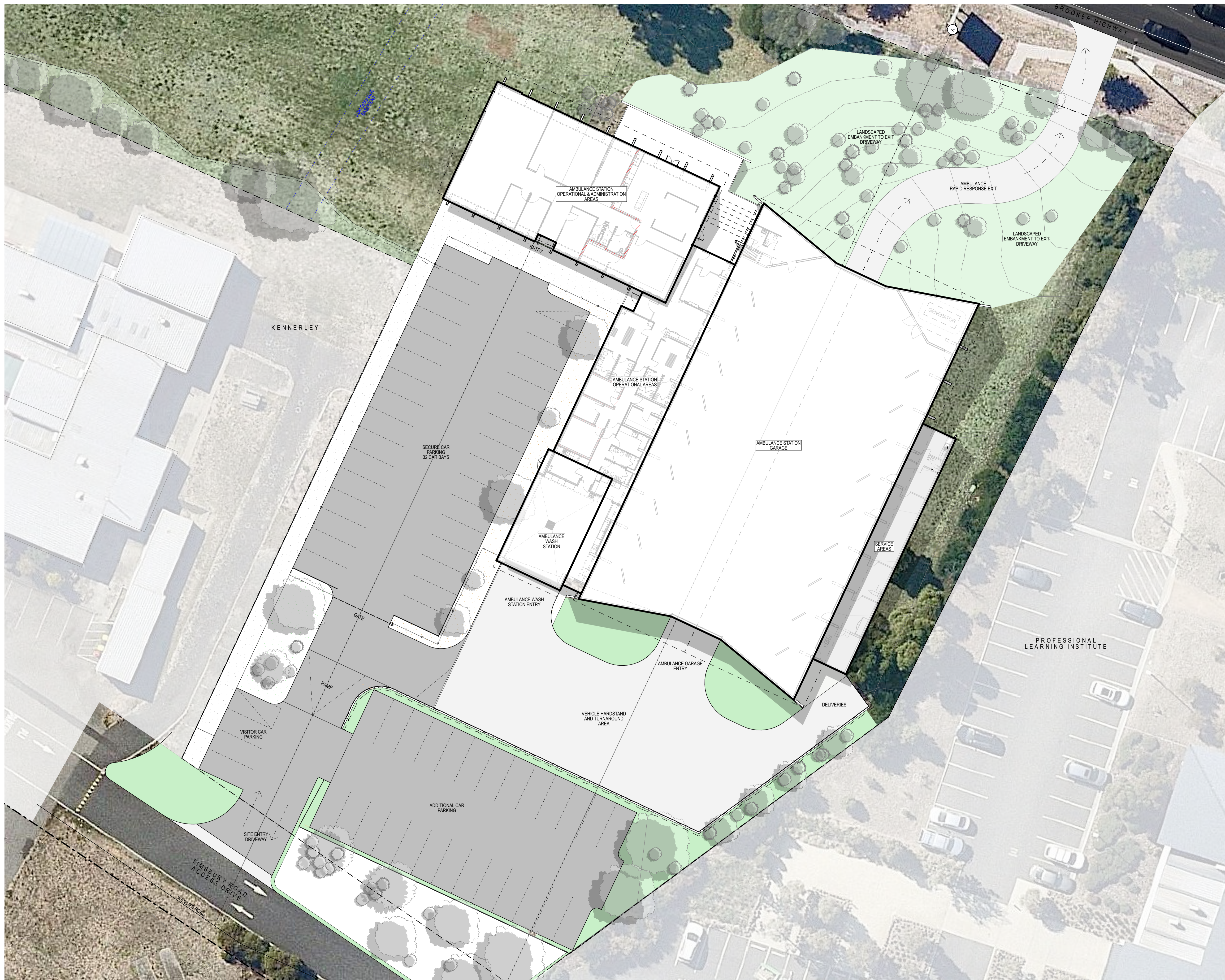
1 SITE PLAN 1:200
